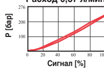
Зависимость давления от уровня сигнала Расход 0,37 л/мин
