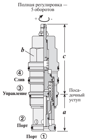
DKDP DKFP DKHP DKJP Открывающее давление
