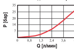
DBAH Зависимость давления от расхода
