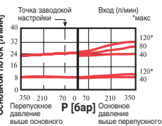
Стандартная диаграмма давления
