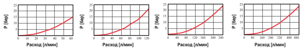
DKDP DKFP DKHP DKJP Открывающее давление
