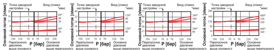
Стандартная диаграмма давления
