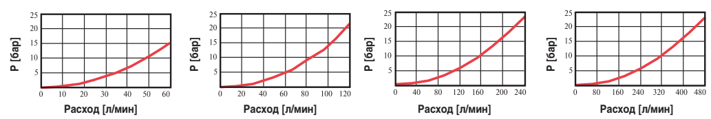
DKDR-8 DKFR-8 DKHR-8 DKJR-8 Открывающее давление
