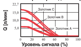
Зависимость расхода от уровня сигнала при перепаде 14 бар
