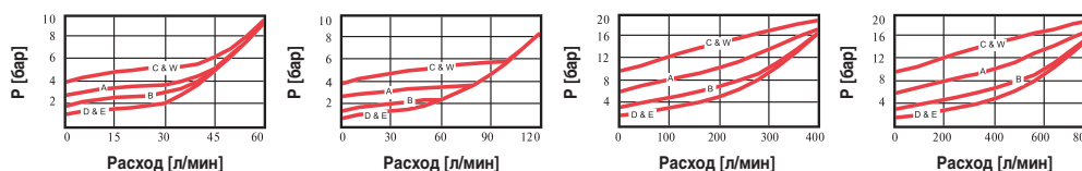
Свободный поток и падение давления при последовательном открытии
