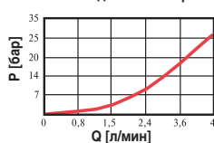
Зависимость давления от расхода
