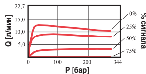
Зависимость расхода от перепада давления
