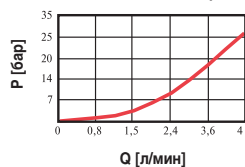
Зависимость давления от расхода
