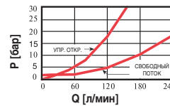
Падение давления при свободном потоке и пилотном давлении
